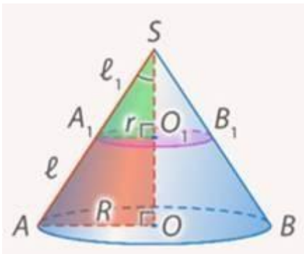
Рис. 14. Подобные треугольники
