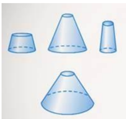
Рис. 2. Геометрические фигуры
